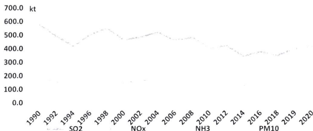
Слика 3.2.10. Емитоване количине примарних суспендованих честица и секундарних прекурсора суспендованих честица у Републици Србији у периоду 1990-2020. године
