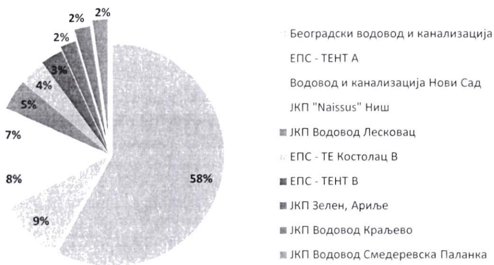
Слика 3.2.18. Највећи извори загађивања емисијом фосфора у Републици Србији у 2021. години
