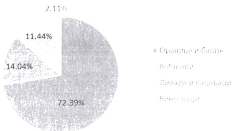
Слика 3.1.41. Процентуални удео узорака према начину коришћења земљишта
