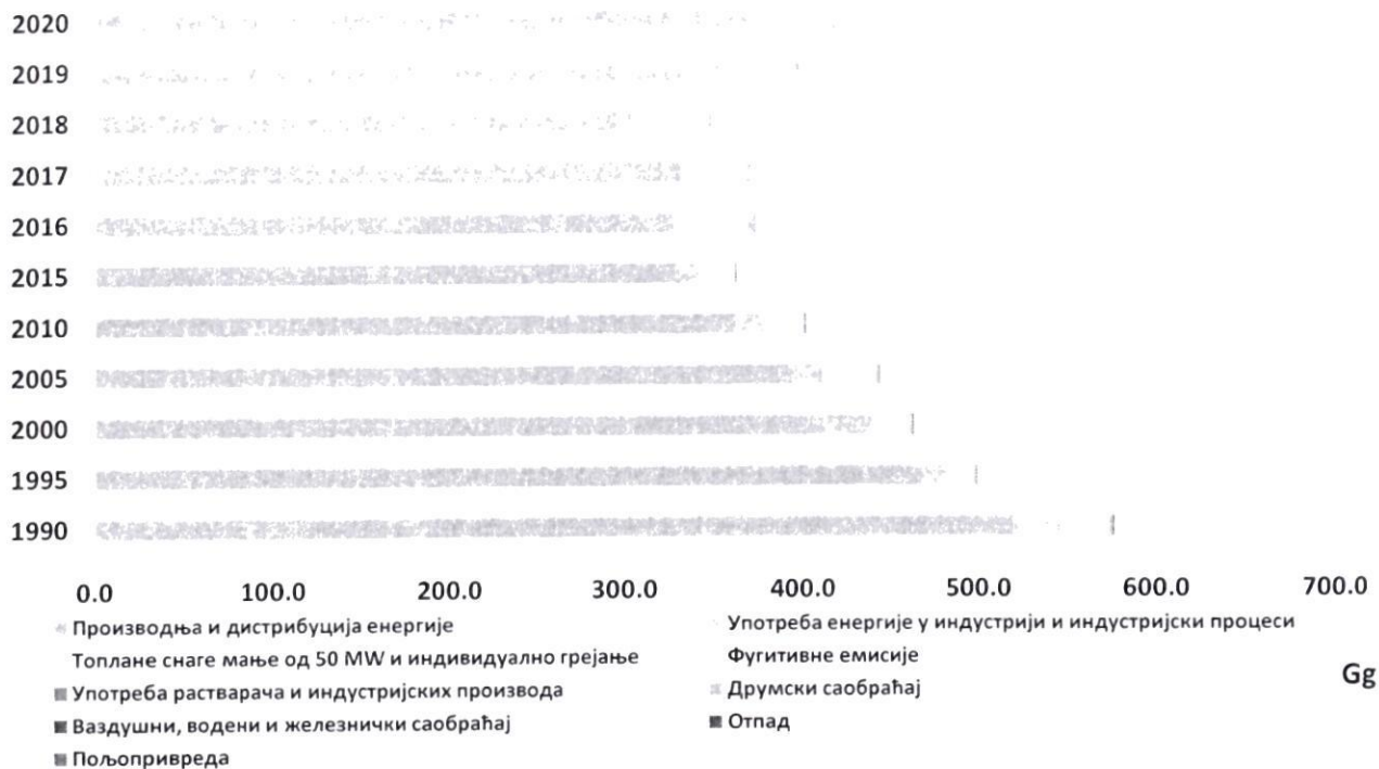
Слика 3.2.5. Емисије сумпорних оксида по секторима у периоду 1990-2020. године изражене у хиљадама тона
