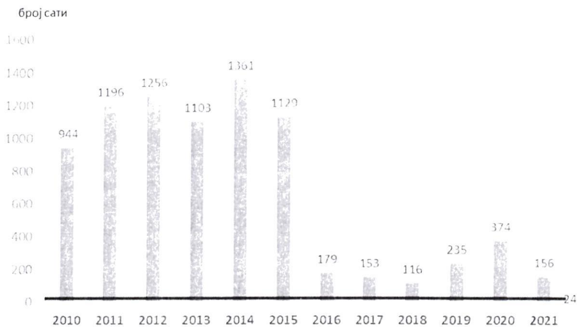
Слика 3.1.6. Број сати током године када је концентрација сумпор диоксида прекорачила граничну вредност ( 350 \mu\text{g}/\text{m}^3 ) на станици Бор Градски парк у периоду 2010-2021. године (дозвољено је 24 сата са прекорачењем током календарске године)
