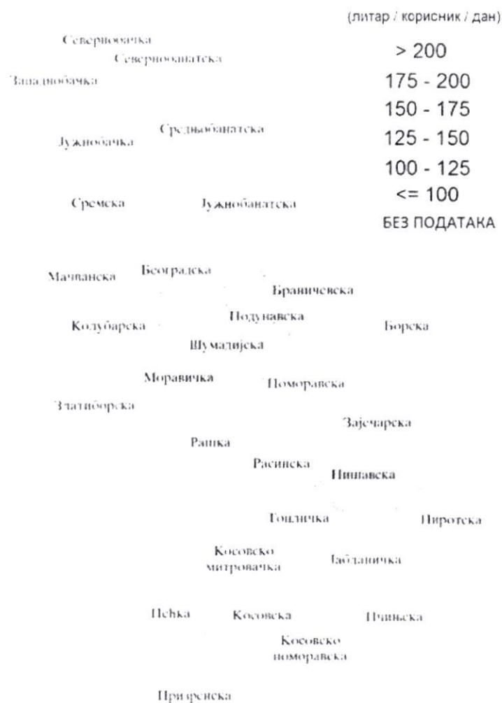
Слика 3.2.24. Коришћење воде у домаћинству по областима Републике Србије (2020. година)
