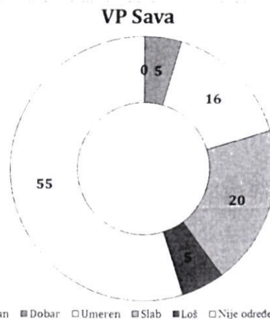
Слика 4.1.2. Еколошки статус водних тела на простору водног подручја Сава (2012-2019)
