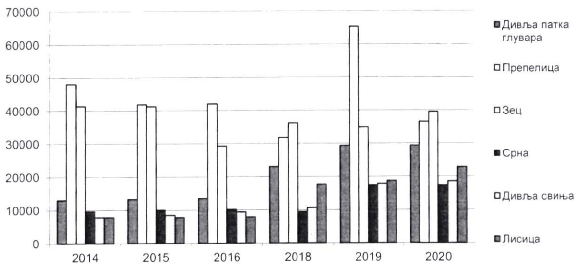
Слика 3.1.58.а. Излов најзначајнијих ловних врста
