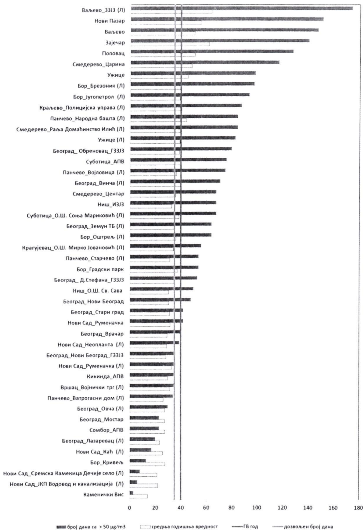
Слика 3.1.10. Средња годишња вредност и број дана са прекораченом дневном граничном вредношћу(50 µg/m³) PM 10 током 2021. године
