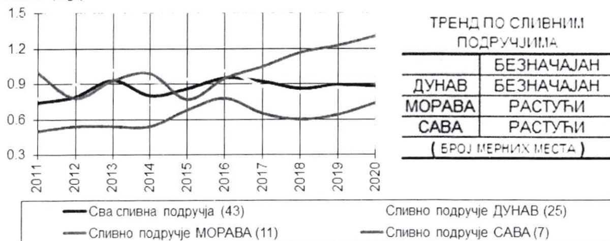
Слика 3.1.20. Трендови медијана нитрата у сливним подручјима Републике Србије (2011-2020. године)
