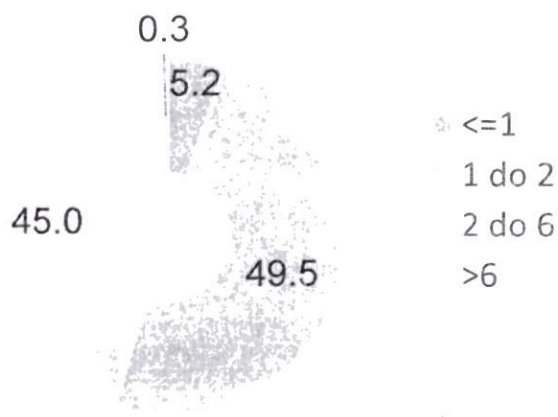
Слика 3.1.46. Удео узорак према садржају органског угљеника у земљишту (%)
