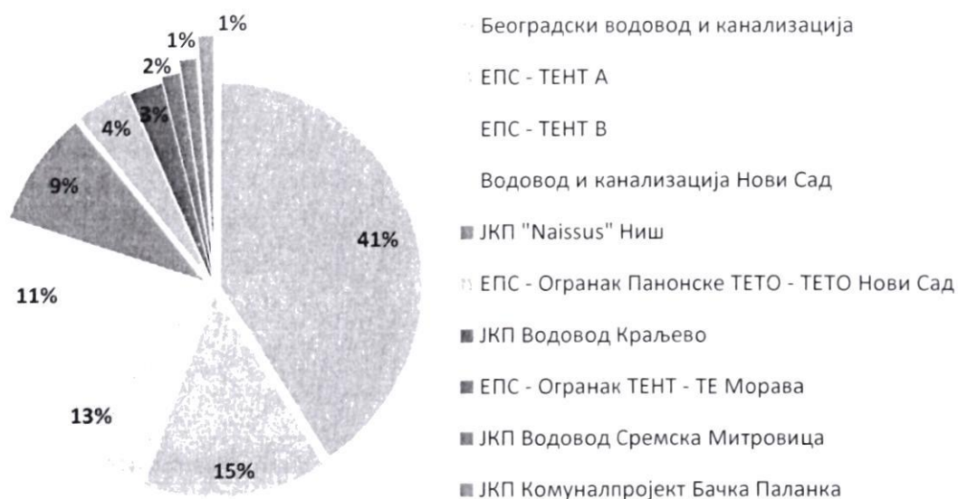
Слика 3.2.17. Највећи извори загађивања емисијом азота у Републици Србији у 2021. години
