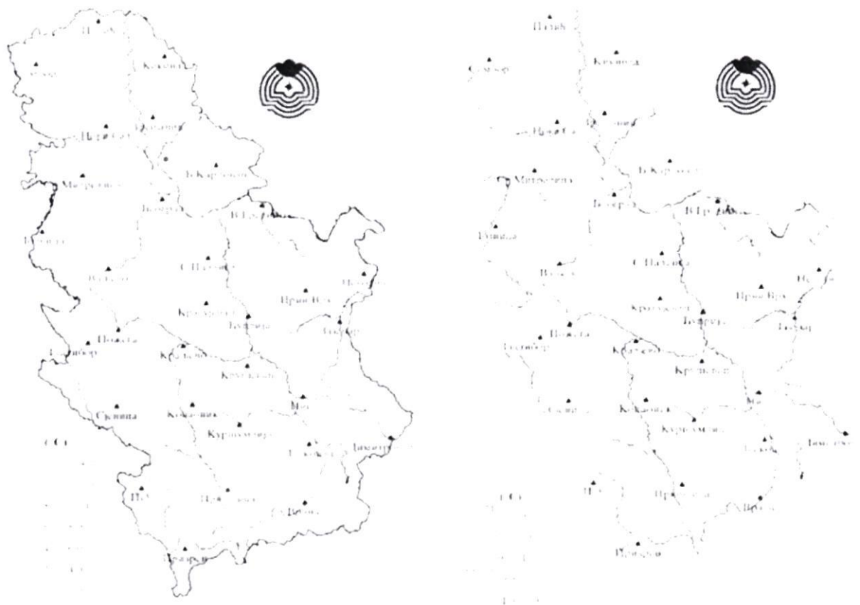
Слика 3.3.11. Распдела годишњих вредности температуре (лево) на подручју Републике Србије у 2021. години и одступања средње годишње температуре у (°C) од нормале 1981-2010. (десно)
