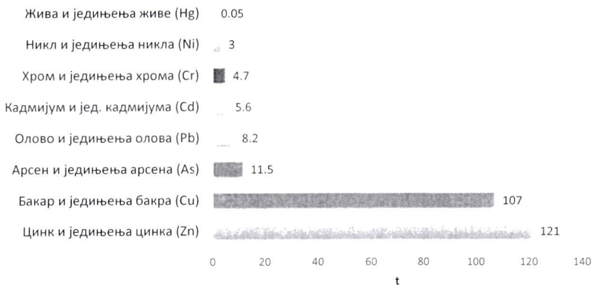
Слика 3.2.22. Емитоване количине тешких метала у отпадним водама у Републици Србији у 2021. години
