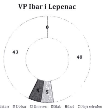
Слика 4.1.4. Еколошки статус водних тела на простору водног подручја Ибар и Лепенац (2012-2019)
