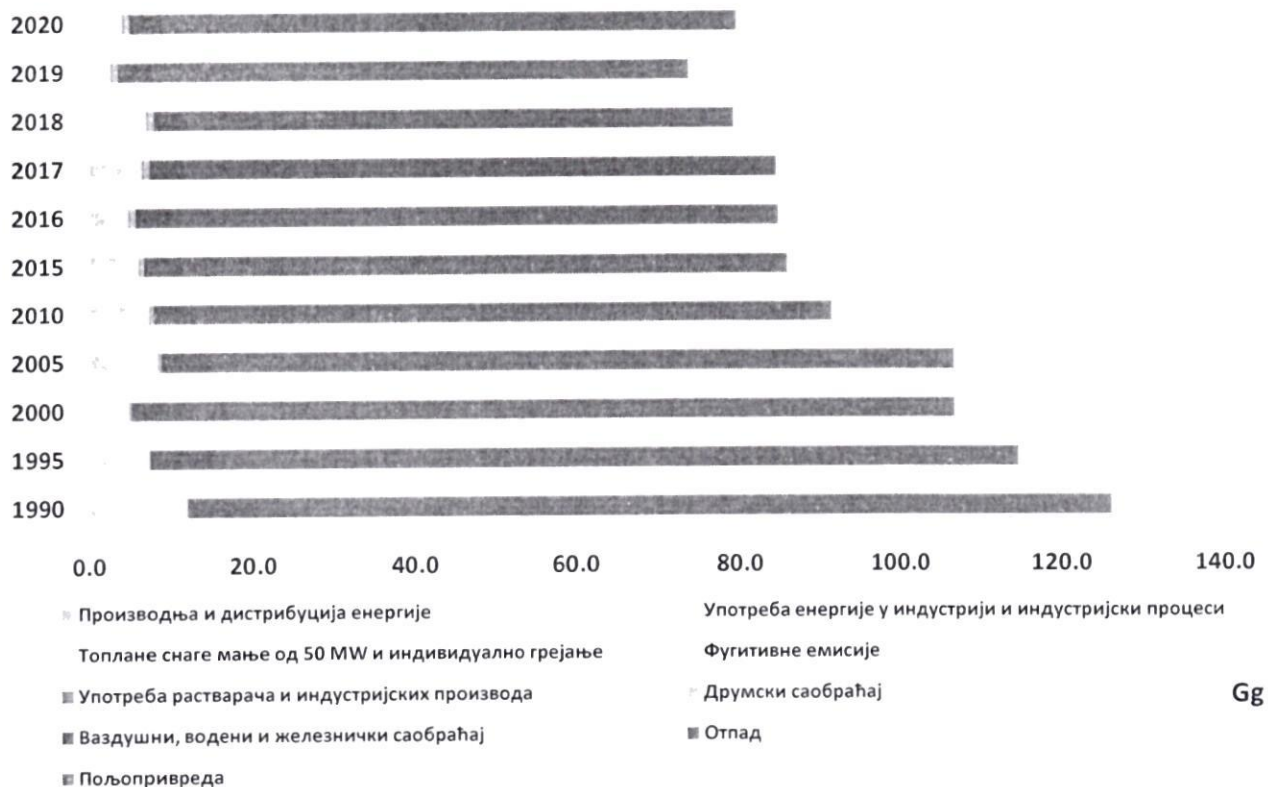
Слика 3.2.6. Емисије амонијака по секторима у периоду 1990-2020. године изражена у хиљадама тона
