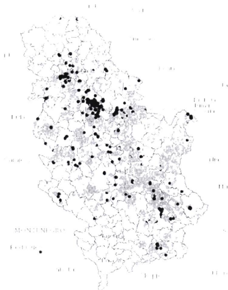
Слика 3.2.35. Дивље депоније на простору Републике Србије
