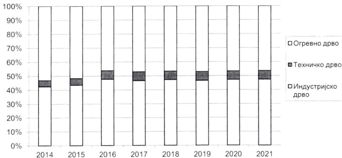
Слика 3.4.10. Структура шумских сортимената из државних шума
