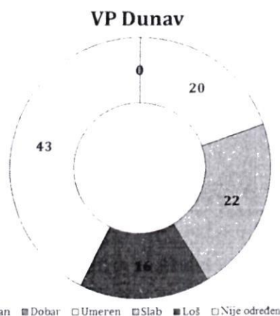
Слика 4.1.1. Еколошки статус водних тела на простору водног подручја Дунав (2012-2019)
