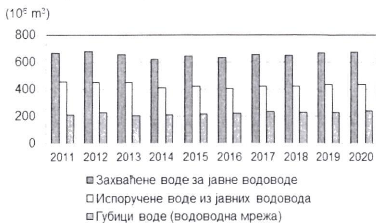
Слика 3.5.20. Ефикасност коришћења вода у водоводима Републике Србије (2011-2020. године)
