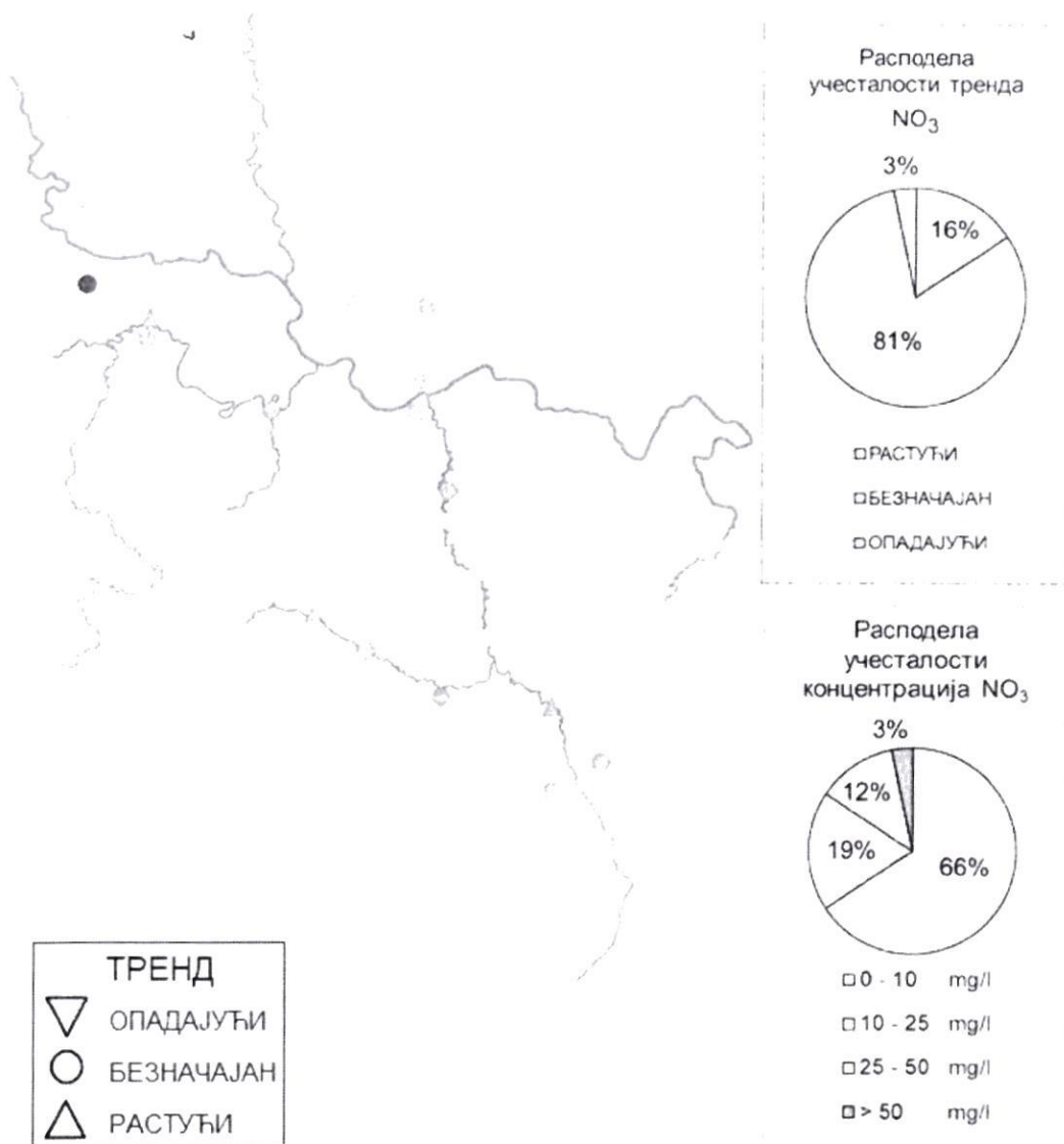
Слика 3.1.36. Тренд и средња вредност концентрација нитрата у подземним водама Републике Србије (2011-2020. године)
