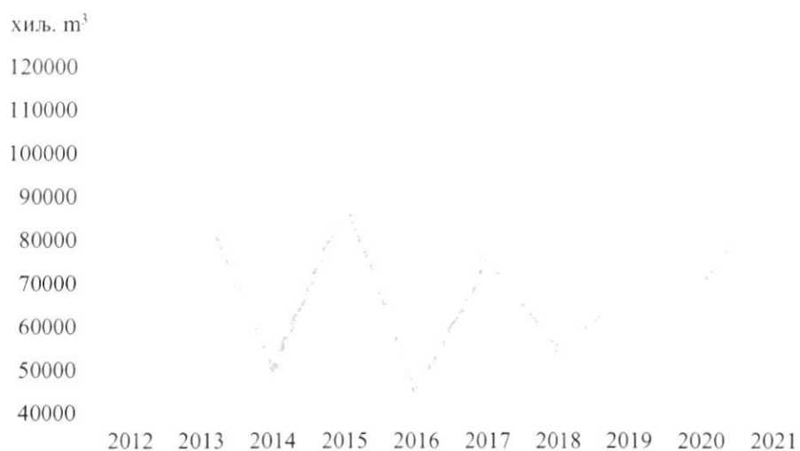
Слика 3.2.43. Захваћене воде за наводњавање пољопривредних површина у Републици Србији у периоду 2012-2021. године (хиљада m³)
