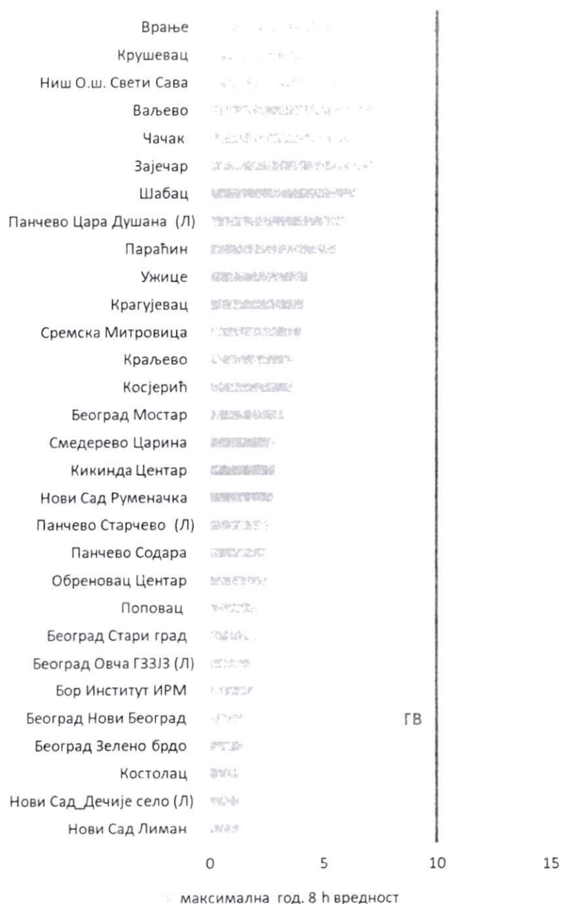
Слика 3.1.17. Приказ максималних осмосатних концентрација угљен монооксида ( \text{mg}/\text{m}^3 ) у 2021. години
