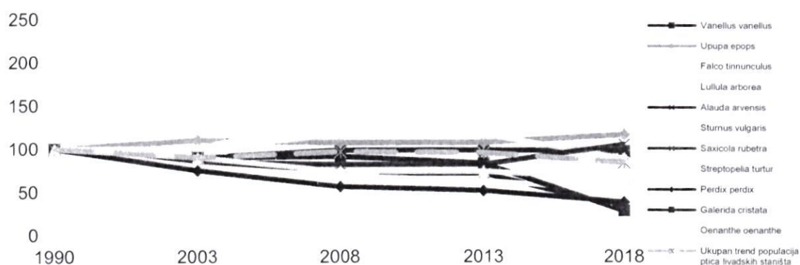
Слика 3.1.49. Тренд популација ливадских врста птица (11 врста)
