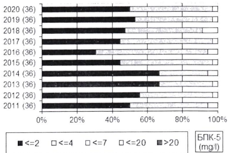
Слика 3.1.28. Распредела учесталости БПК-5 у водотоцима Републике Србије (2011-2020. године)
