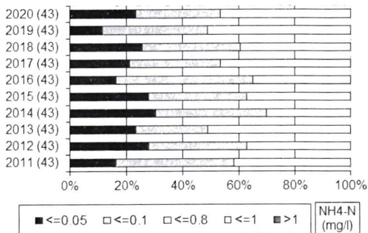
Слика 3.1.31. Расподела учесталости амонијума у водотоцима Републике Србије (2011-2020. године)
