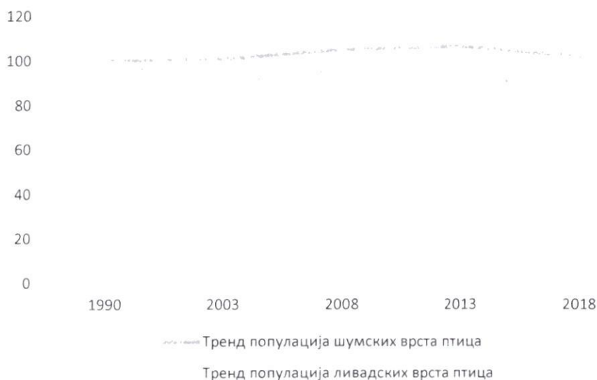
Слика 3.1.48. Тренд популација птица у Републици Србији
