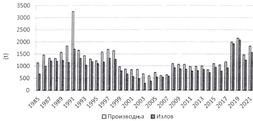
Слика 3.4.16. Производња и излов у пастрмским рибањацима
