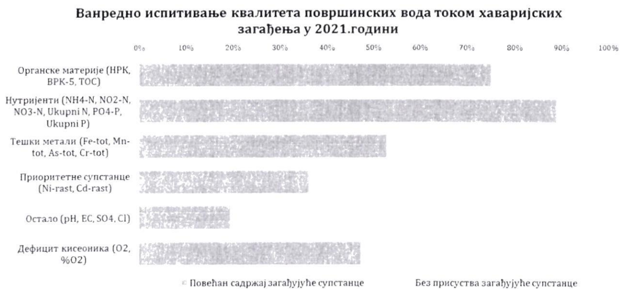
Слика 2.3. Загађујуће материје присутне у води водотока након хаваријских загађења у 2021. години
