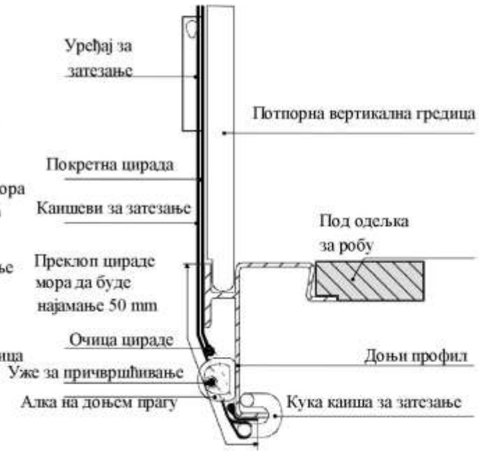
Цртеж бр.9.3 ПРЕКЛОП ЦИРАДЕ НА ДНУ ВОЗИЛА
